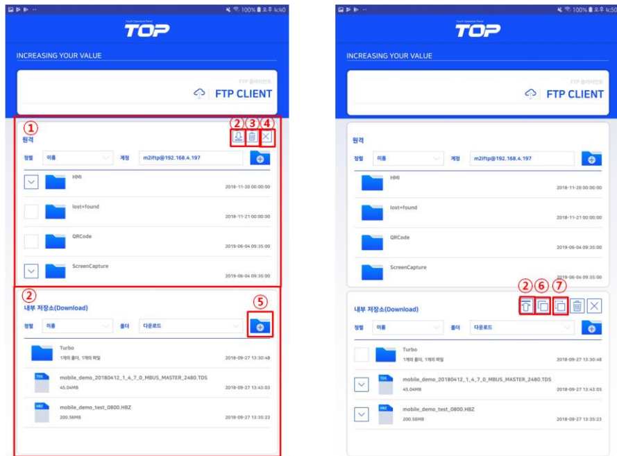
[그림. 13] FTP 클라이언트 화면
