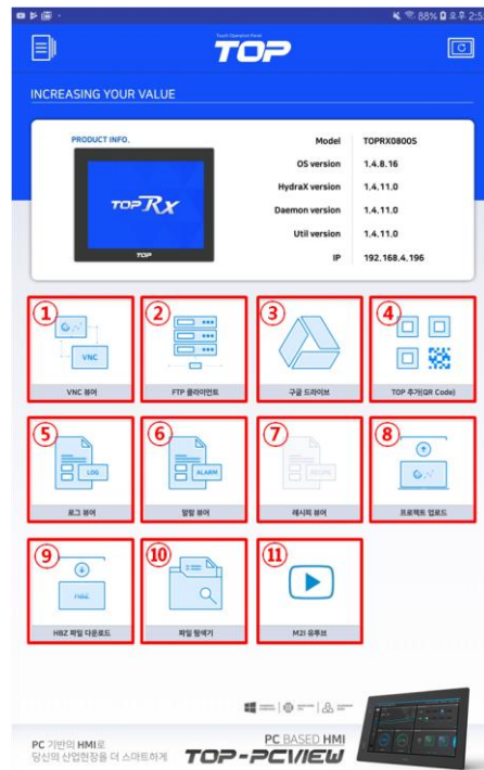
[그림. 11] TOP TOOLS 기능
